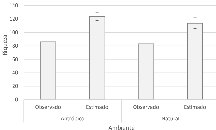
Figura 269 Relação das riquezas de espécies observadas e estimadas para os tipos de habitats amostrados
