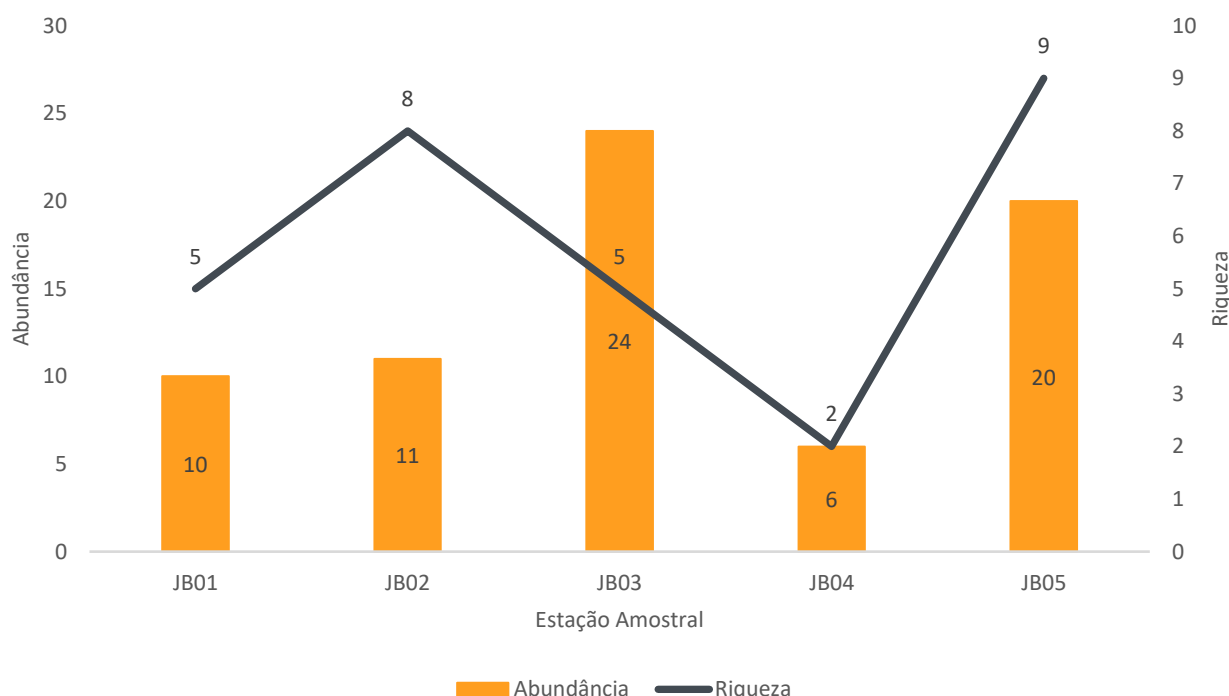
Figura 97 Riqueza e abundância de besouros registrada em cada estação amostral durante o levantamento
