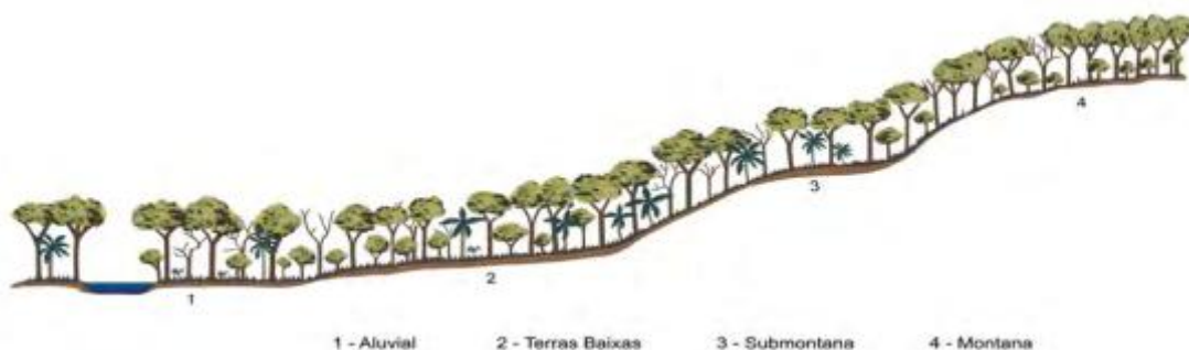
Figura 02 Perfil esquemático da Floresta Estacional Semidecidual
