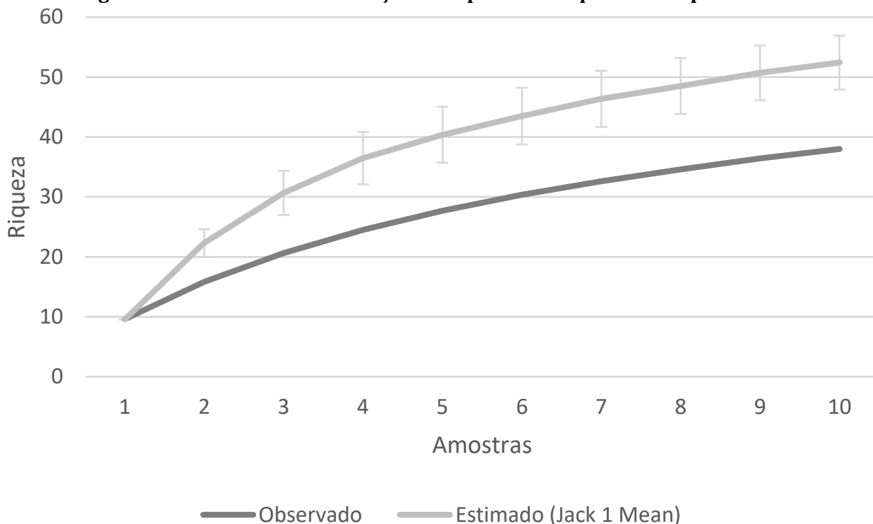
Figura 82 Curva de acumulação de espécies de dípteras com potencial vetor
