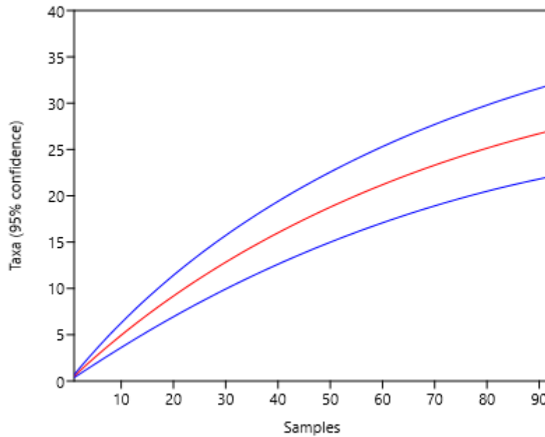
Figura 389 Curva de rarefação de espécies de mamíferos no estudo
