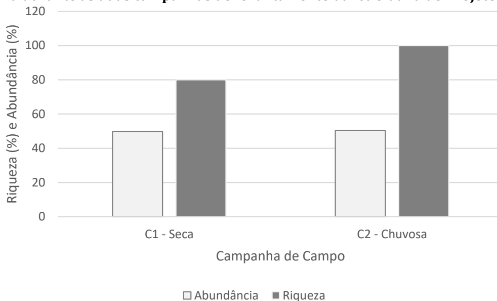
Figura 128 Abundância e riqueza de espécies da ictiofauna registradas nos períodos de seca e chuva durante as duas campanhas do levantamento da ictiofauna do Projeto Jambreiro
