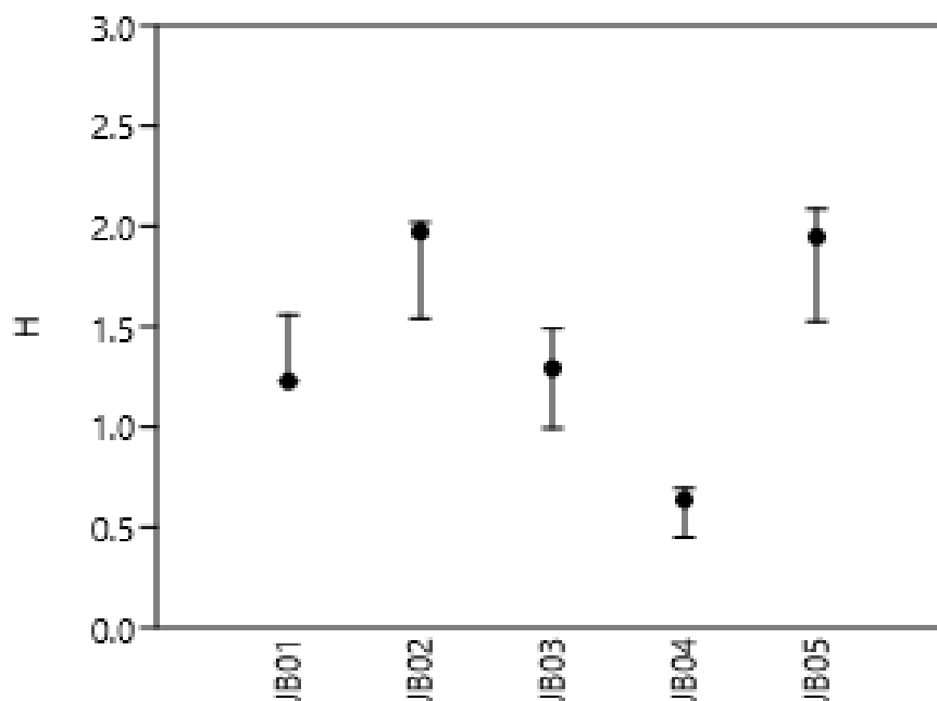
Figura 99 Variação de shannon e do índice de confiança em cada estação amostral do levantamento de besouros
