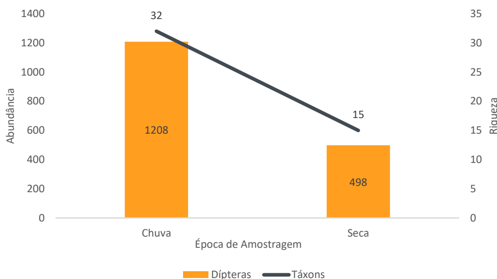
Figura 74 Riqueza e Abundância de dípteras registrada em cada campanha do levantamento
