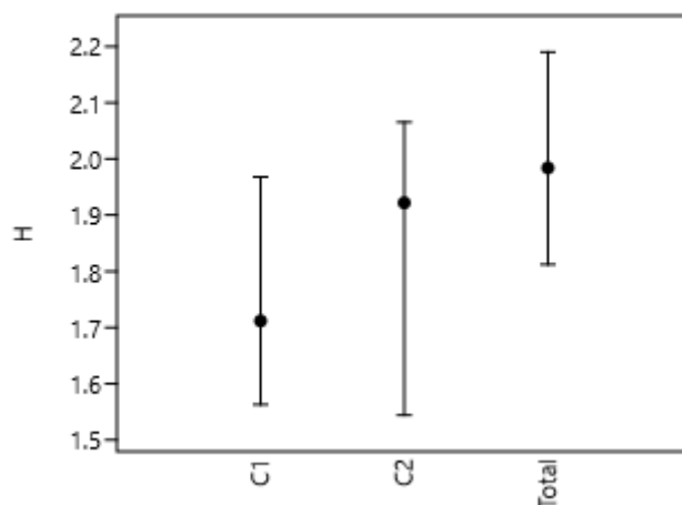
Figura 95 Índice de shannon e bootstrap 95% de escarabeíneos registrados em cada campanha do levantamento.
