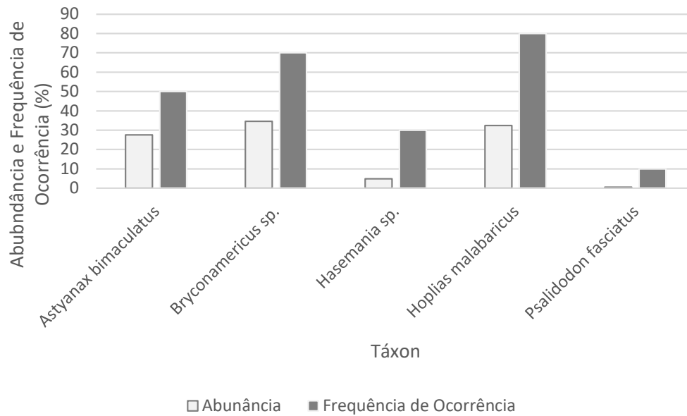
Figura 124 Abundância e frequência de ocorrência das espécies registradas durante as duas campanhas do levantamento da ictiofauna do Projeto Jambreiro
