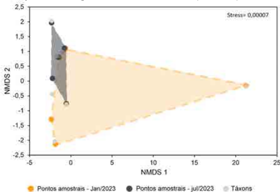
Figura 157 Análise espacial NMDS da distribuição da comunidade de Macroinvertebrados bentônicos de acordo a dissimilaridade entre os pontos de amostragens pela distância de “Bray-Curtis” nos períodos chuvoso e seco de janeiro e julho de 2023
