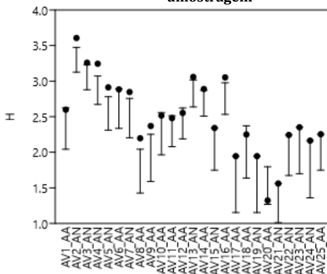
Figura 271 Índice de shannon e bootstrap 95% de aves registrada em cada unidade de amostragem
