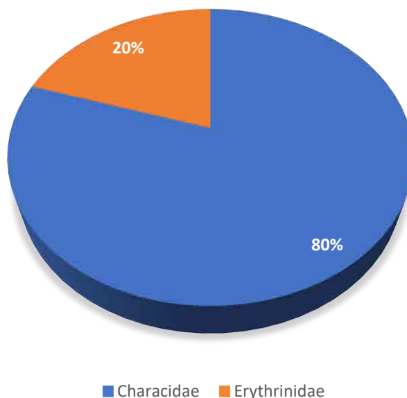
Figura 123 Percentual de espécies por Famílias registradas durante as duas campanhas do Levantamento da ictiofauna do Projeto Jambreiro
