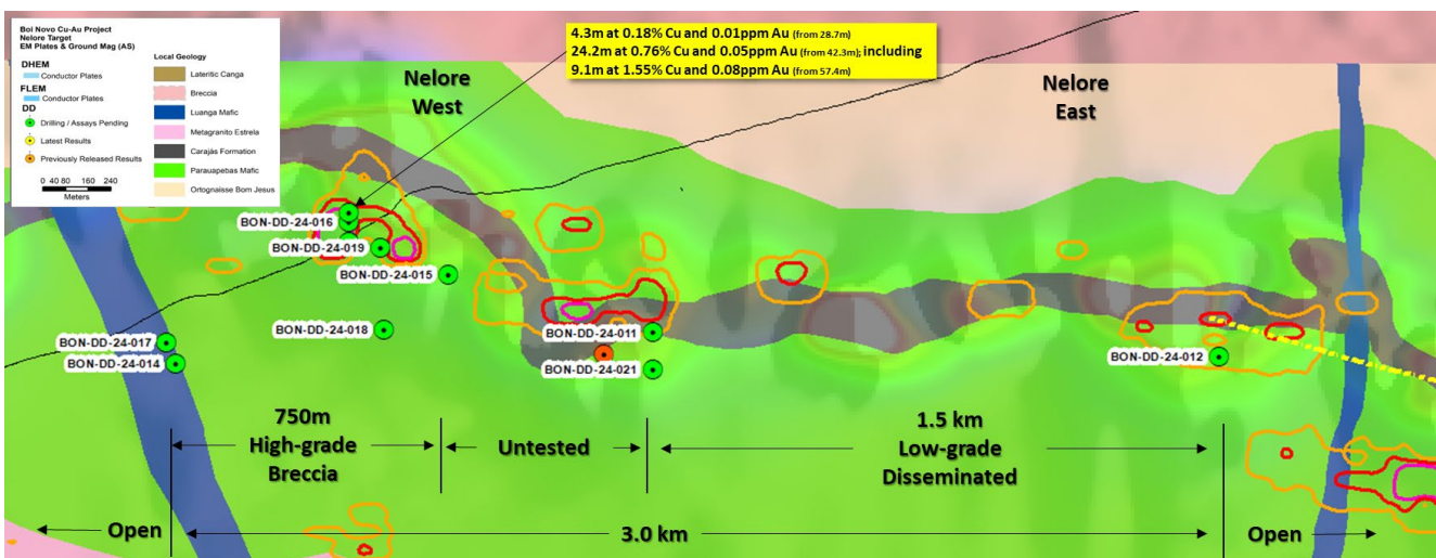
Figure 3 – Nelore Prospect Plan Map.
